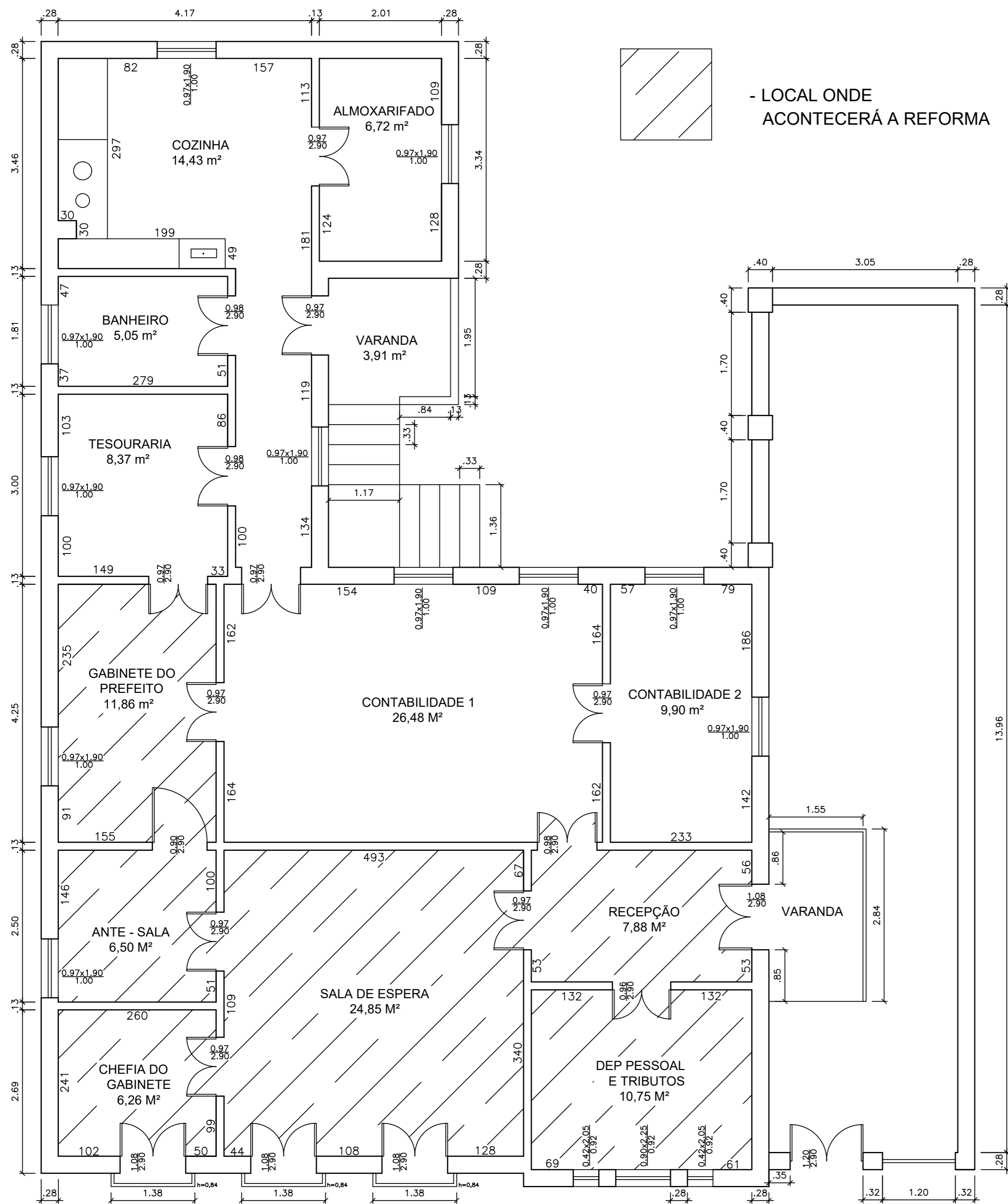
PLANTA BAIXA ESC: 1/50
